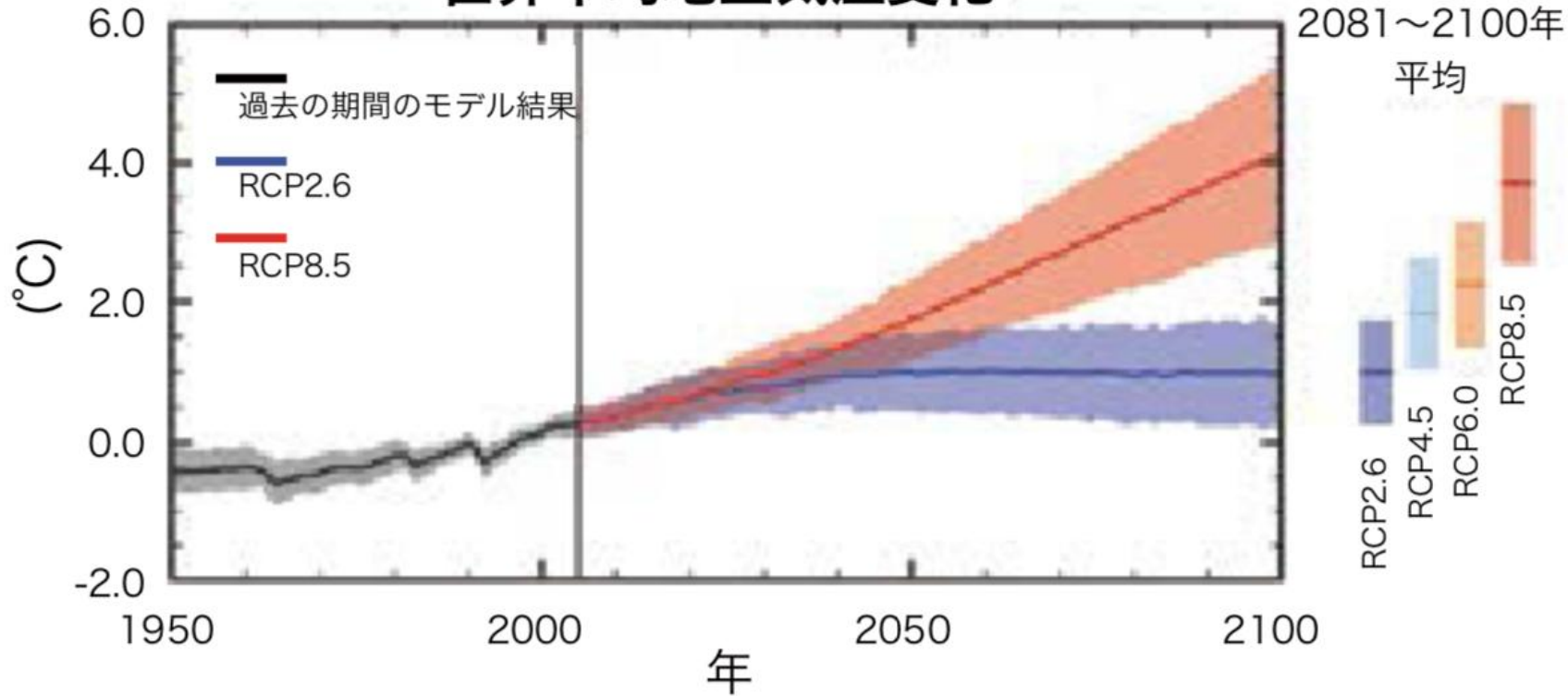
世界平均地上気温変化
